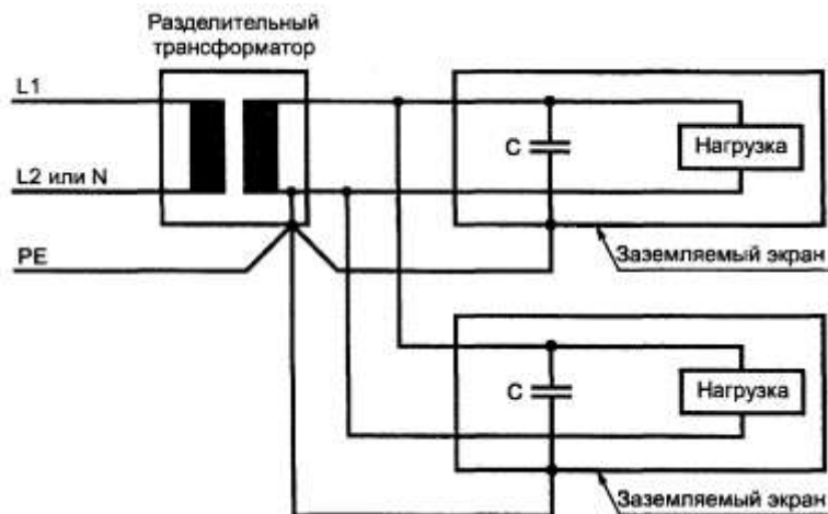
Рисунок А.1 — Границы между электроустановкой и оборудованием обработки информации
