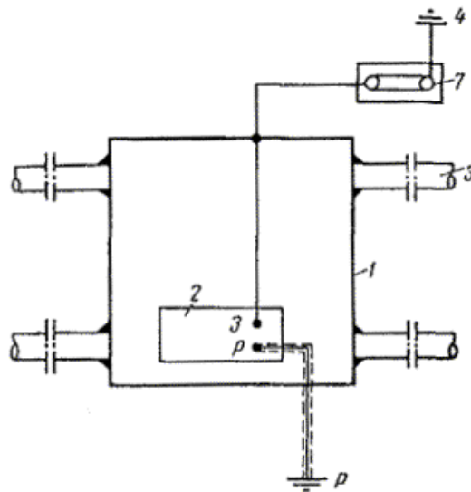
Рис. 11.9. Ввод и заземление кабелей без изолирующего покрытия ( r_3 > 300 \text{ Ом*м} )
