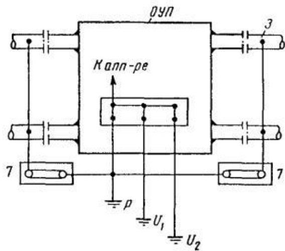
Рис. 11.10. Ввод в ОУП и заземление кабелей без изолирующего покрытия U_1 , U_2 - первое и второе измерительные напряжения соответственно
