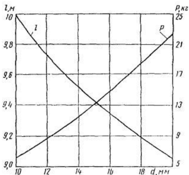
Рис.2.16. Зависимости веса и длины глубинного заземлителя от диаметра стержня при постоянном сопротивлении заземления
