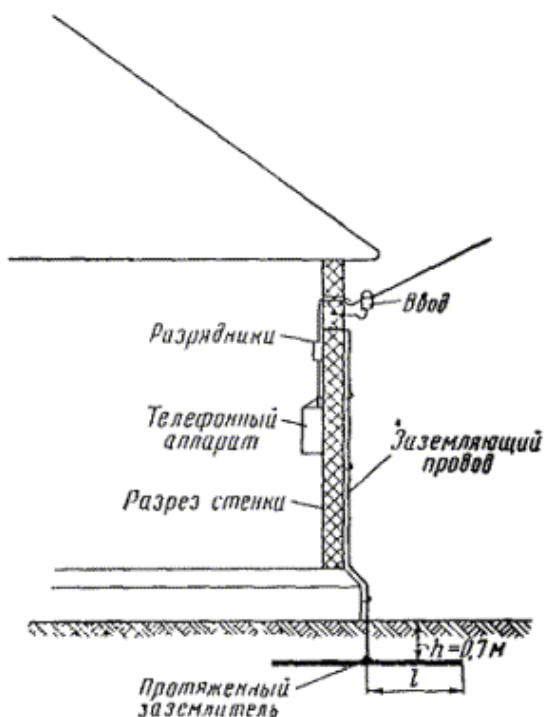
Рис. 4.1. Устройство заземления с использованием в качестве заземлителя водопроводной трубы
