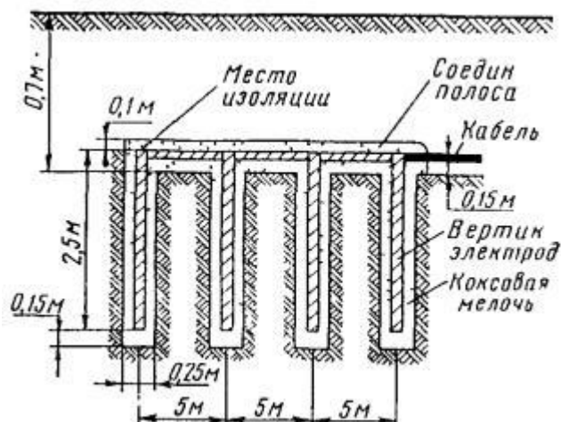
Рис.2.19 Схема установки многоэлектродного заземления в коксовой засыпке
