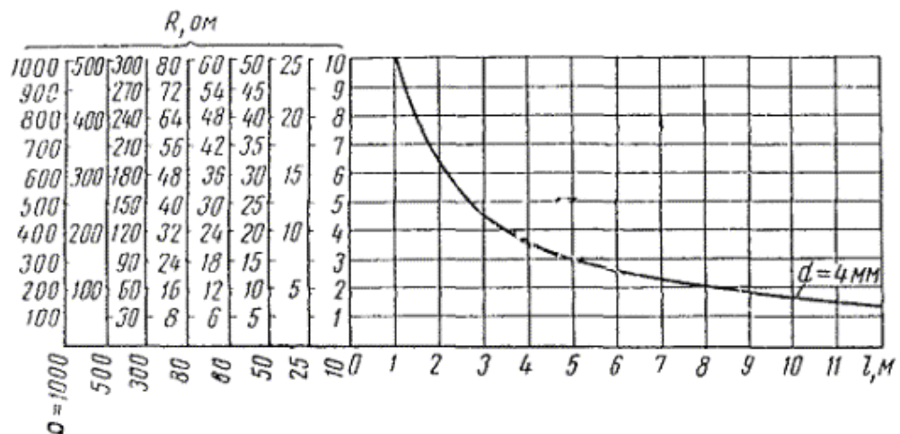
Рис.2.8. Кривая изменения сопротивления кольцевого заземлителя в зависимости от радиуса кольца при d=4 мм, глубине заковки заземлителя h = 0,5 - 0,7 м для различных значений удельного сопротивления грунта
