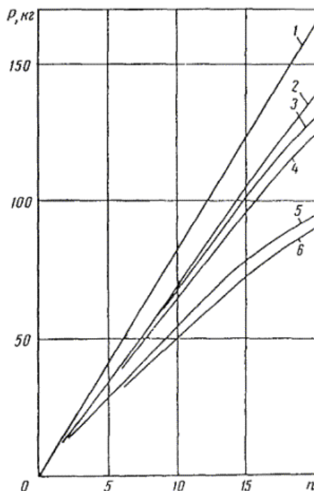
Рис.2.14. Вес многоэлектродного и глубинного заземлений при одинаковом сопротивлении в однородном грунте: 1 - вес многоэлектродного заземления в зависимости от количества электродов; 2 - вес эквивалентного глубинного заземления при выполнении многоэлектродного заземления в виде контура с расстоянием между электродами 7,5 м; 3 - вес эквивалентного глубинного заземлителя при выполнении многоэлектродного заземления в виде ряда с расстоянием между электродами 5 м; 4 - вес эквивалентного глубинного заземлителя при выполнении многоэлектродного заземления в виде контура с расстоянием между электродами 5 м; 5 - вес эквивалентного глубинного заземлителя при выполнении многоэлектродного заземления в виде ряда с расстоянием между электродами 2,5 м; 6 - вес эквивалентного глубинного заземлителя при выполнении многоэлектродного заземления в виде много электродного замкнутого контура с расстоянием между электродами 2,5 м
