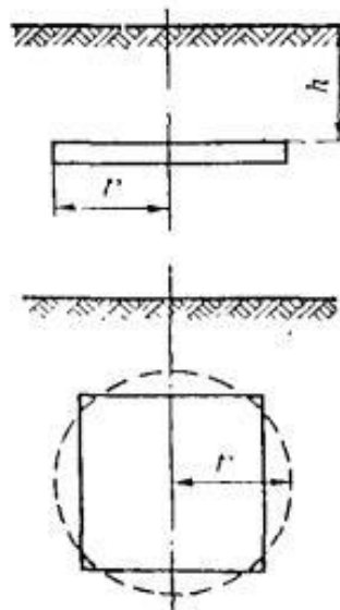
Рис.2.9. Пластинчатый заземлитель
