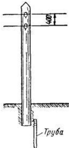
Рис. 3.6. Опора с заземлением из одной трубы
