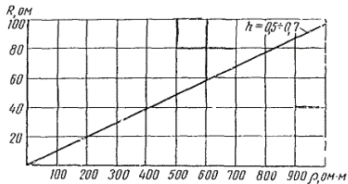
Рис.2.10. График изменения сопротивления пластинчатых заземлителей в зависимости от удельного сопротивления грунта для пластины с эквивалентным радиусом, равным 0,55 м, при h = 0,5 - 0,7 м
