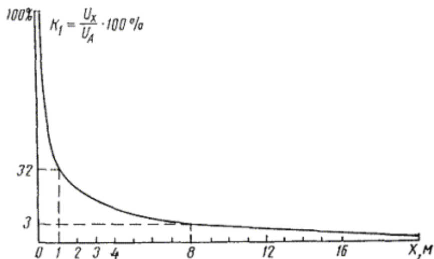
Рис.1.2. Кривая изменения отношения \kappa_1 потенциала точек земли между двумя заземлителями U_x к потенциалу заземлителя относительно нулевой точки в зависимости от расстояния x
