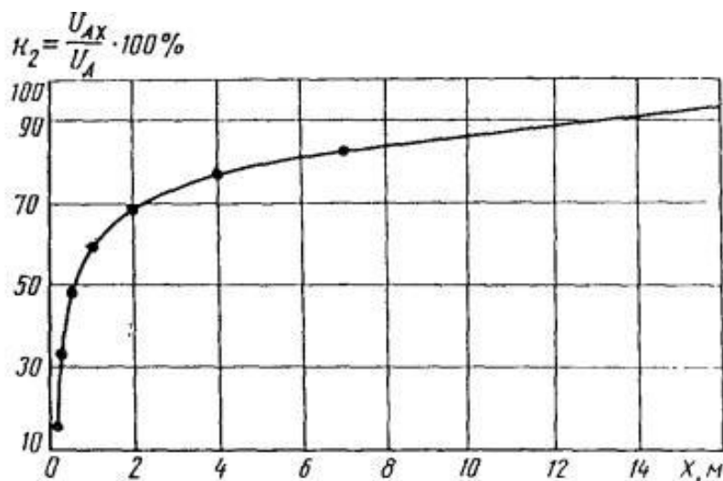
Рис. 1.3. Кривая изменения отношения \kappa_2 (в процентах) разности потенциалов U_{Ax} между заземлителем и рассматриваемой точкой x к потенциалу заземлителя U_A в зависимости от расстояния x
