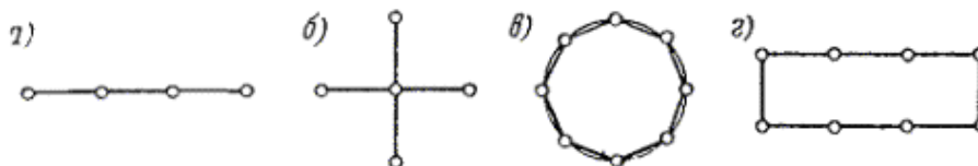
Рис.3.8 Расположение трубчатых заземлителей при устройстве многоэлектродных заземлений а) в ряд; б) в форме креста; в) в форме круга, г) в форме прямоугольника
