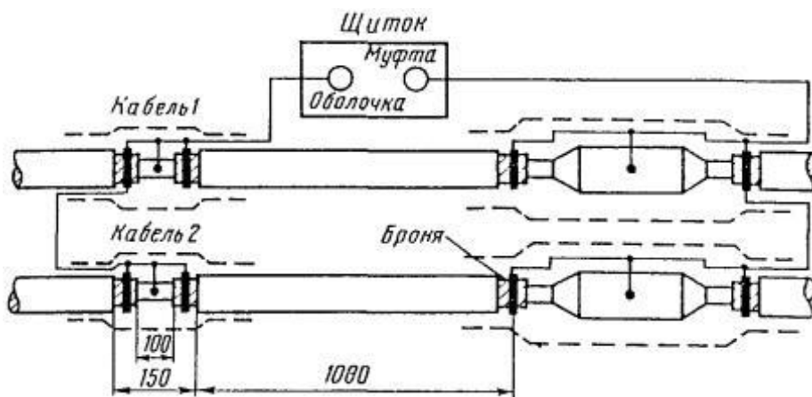
Рис. 11.1. Схема соединений КИП-1 для бронированных кабелей без изолирующих покровов
