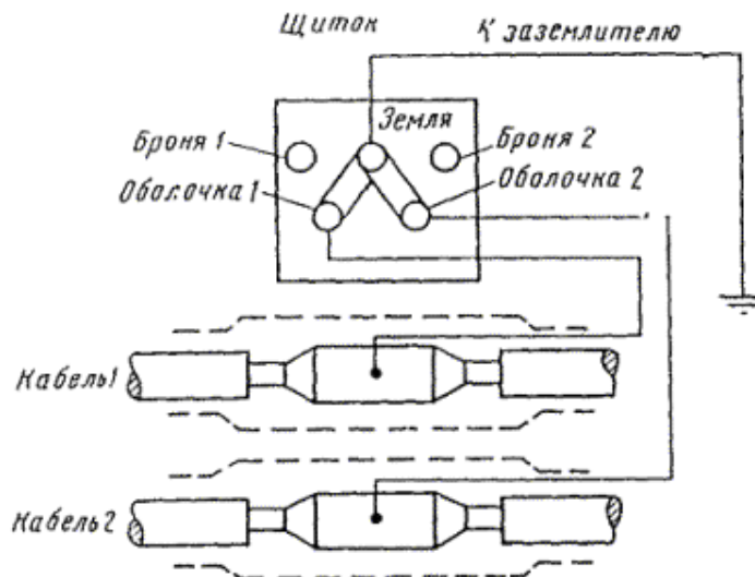
Рис. 11.3. Схема соединений КИП-2 для небронированных кабелей с изолирующим покровом
