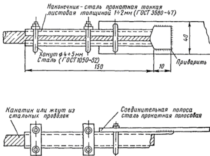
Рис. 5.2. Присоединение подводящего канатика или жгута из проволок к соединительной полосе
