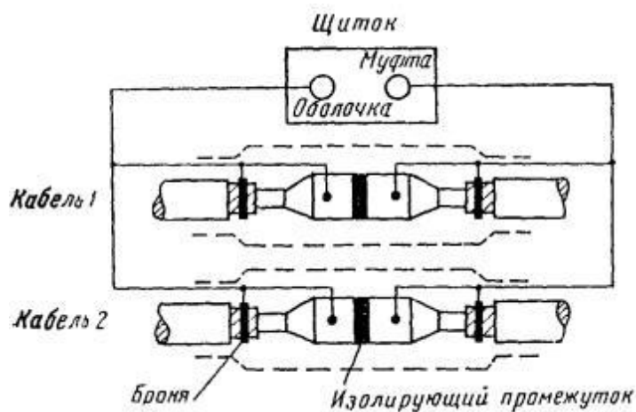
Рис.11.4. Схема соединений КИП-1 при установке изолирующих муфт на бронированных кабелях без изолирующих покровов
