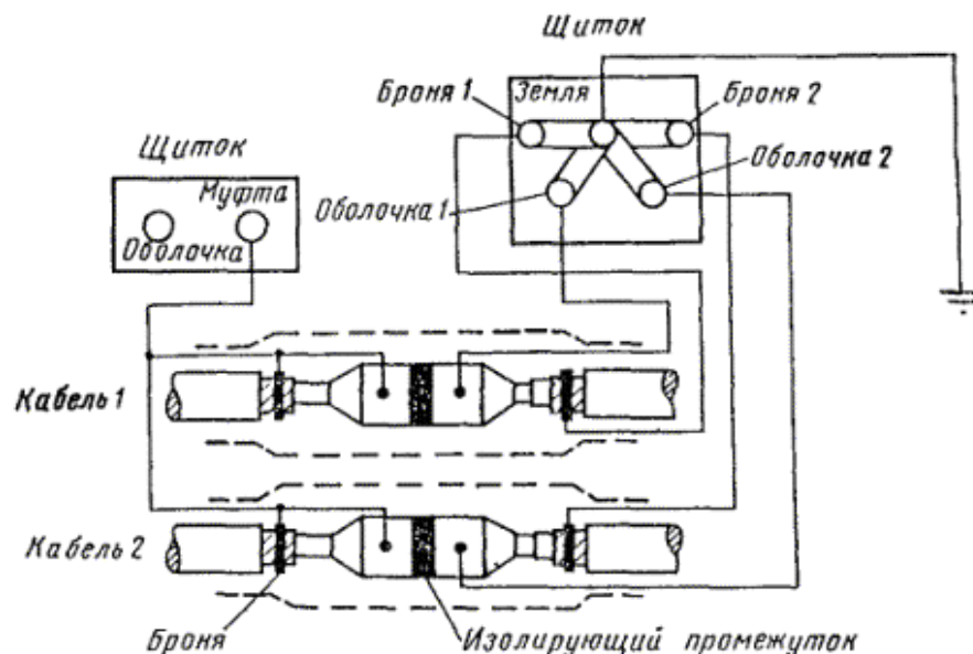
Рис. 11.5. Схема соединений КИП-1 и КИП-2 при установке изолирующих муфт между бронированным кабелем без изолирующих покровов и бронированным кабелем с изолирующим покровом
