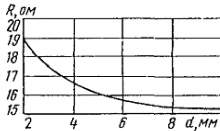
Рис 2.6. Кривая изменения сопротивления протяженного проволочного заземлителя в зависимости от диаметра его проволочек
