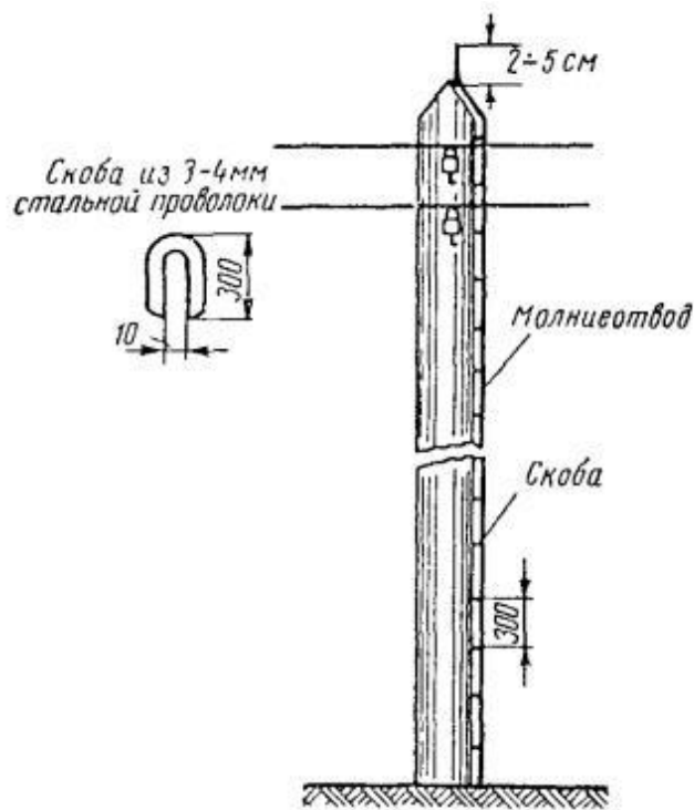
Рис 3.1 Устройство молниеотвода на опоре (молниеотвод крепится скобами вплотную к столбу)
