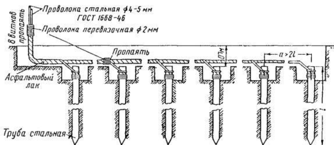
Рис. 3.10. Соединение трубчатых заземлителей проводами
