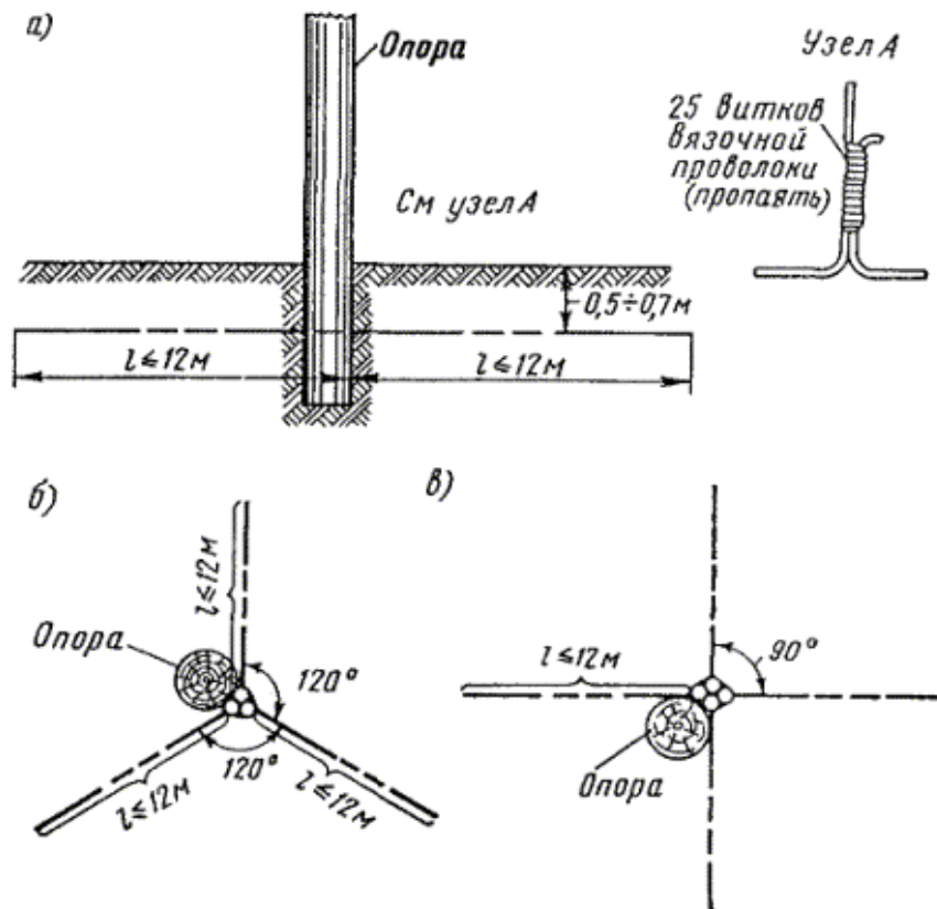
Рис.3.5. Заземление молниеотвода в виде горизонтальных лучей: а) двухлучевого; б) трехлучевого; в) четырехлучевого
