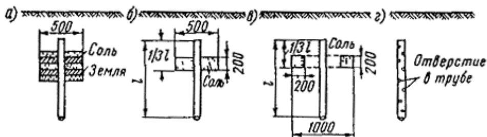
Рис.2.23 Способы укладки соли около вертикального заземлителя
