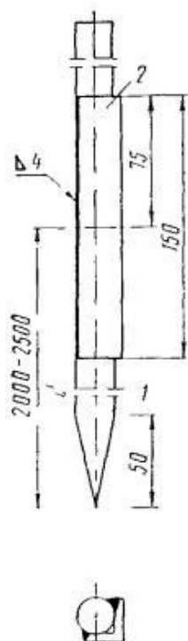
Рис.3.12. Сварка секций глубинных заземлителей с помощью отрезка уголка
