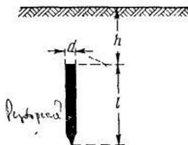
Рис. 2.3. Трубчатый заземлитель
