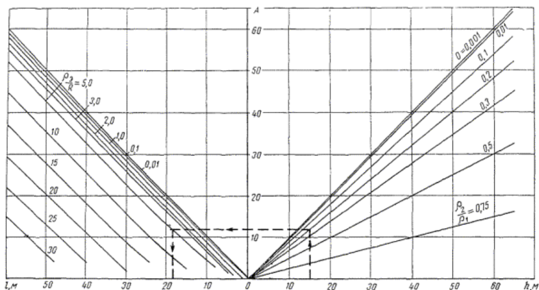
Рис. 2.15 Номограмма для определения длины глубинного заземлителя
