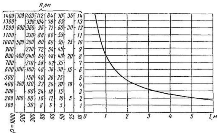
Рис. 2.7. Кривая изменения сопротивления протяженного проволочного заземлителя в зависимости от его длины при d = 4 мм и глубине заделки h = 0,5 - 0,7 м для различных значений удельного сопротивления грунта
