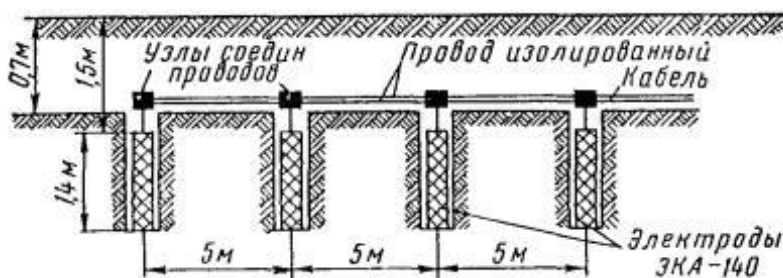
Рис 2.20. Схема установки многоэлектродного заземления из электродов типа ЗКА-140
