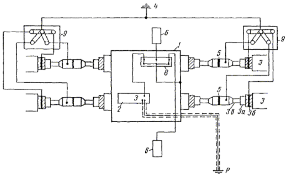
Рис. 11.7. Ввод в НУП и заземление кабелей с изолирующим покрытием ( r_3 = 300 \text{ Ом*м} )
