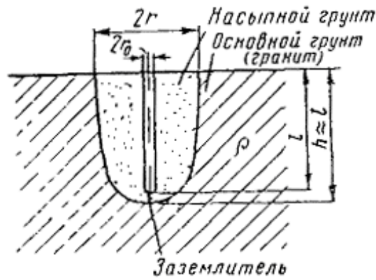
Рис.2.21 Создание вокруг заземлителя зоны с пониженным удельным сопротивлением
