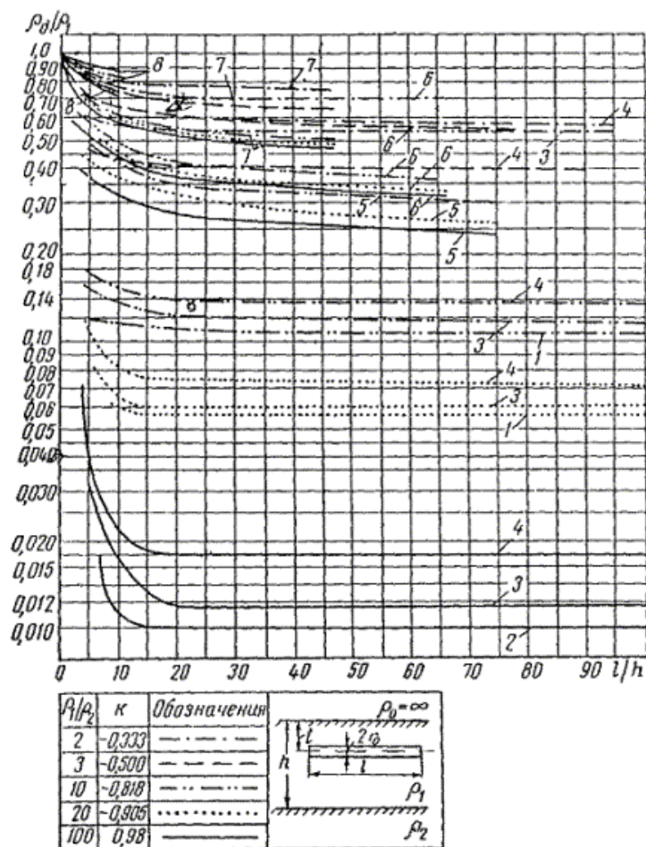
Рис.2.13. Графики действующего удельного сопротивления грунта для горизонтальных заземлителей при различных отношениях t/h и \kappa < 0 :
