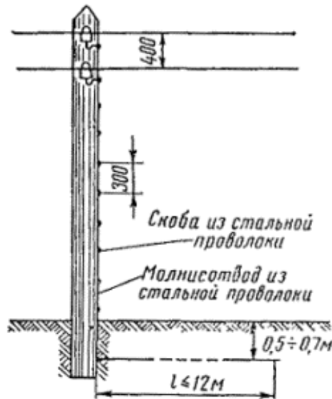
Рис. 3.4. Заземление молниеотвода в виде горизонтального луча
