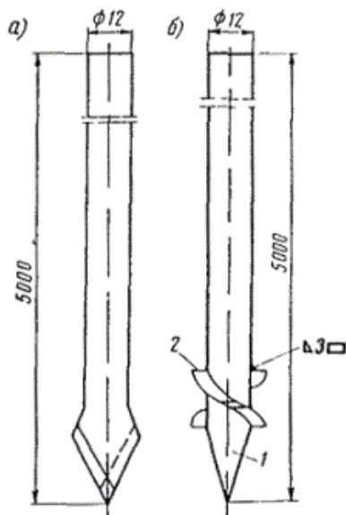
Рис. 3.11. Нижний конец прутка при ввертывании глубинных заземлителей
