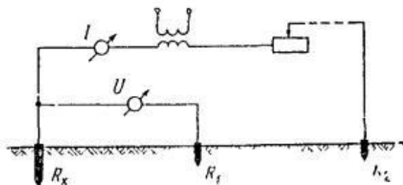
Рис. 8.7 Схема измерения сопротивления заземления с помощью амперметра - вольтметра
