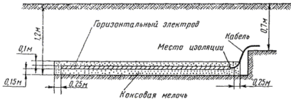
Рис.2.18. Схема установки одиночного горизонтального заземлителя в коксовой засыпке
