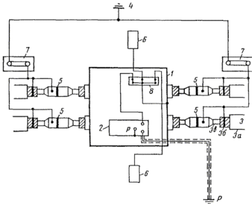
Рис.11.6. Ввод в НУП и заземление кабелей без изолирующего покрытия (удельное сопротивление земли < 300 \text{ Ом*м} ):
