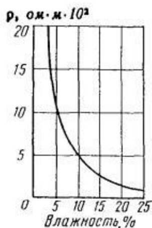
Рис. 2.1. Кривая изменения удельного сопротивления красной глины в зависимости от ее влажности
