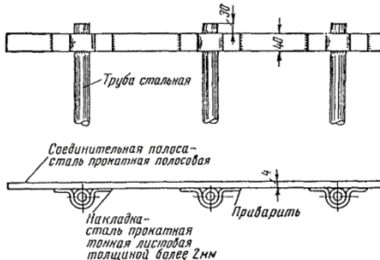
Рис.5.1. Соединение стальной полосой трубчатых заземлителей после забивки их в грунт
