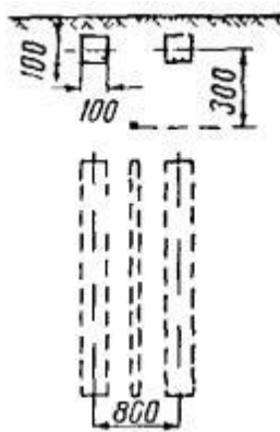
Рис 2.24 Укладка соли около протяженного горизонтального заземлителя
