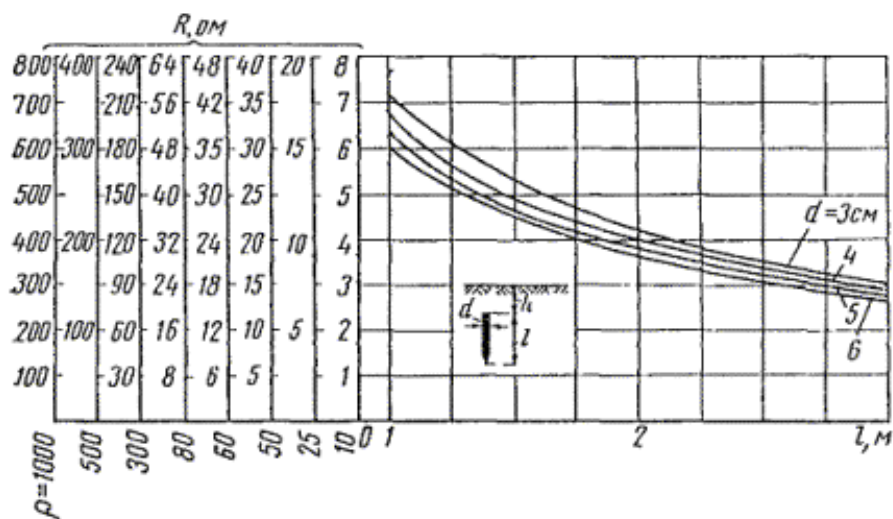
Рис. 2.4. Кривые изменения сопротивления R_a трубчатого заземлителя в зависимости от его длины l при различных диаметрах труб d и различных удельных сопротивлениях \rho грунта (при глубине закопки заземлителя, равной 0,7 м)
