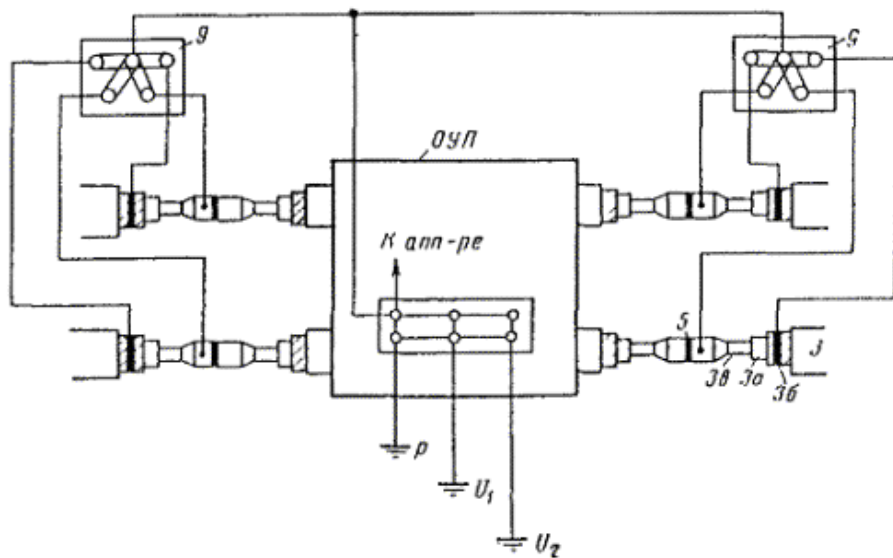
Рис. 11.11. Ввод в ОУП и заземление кабелей с изолирующим покрытием
