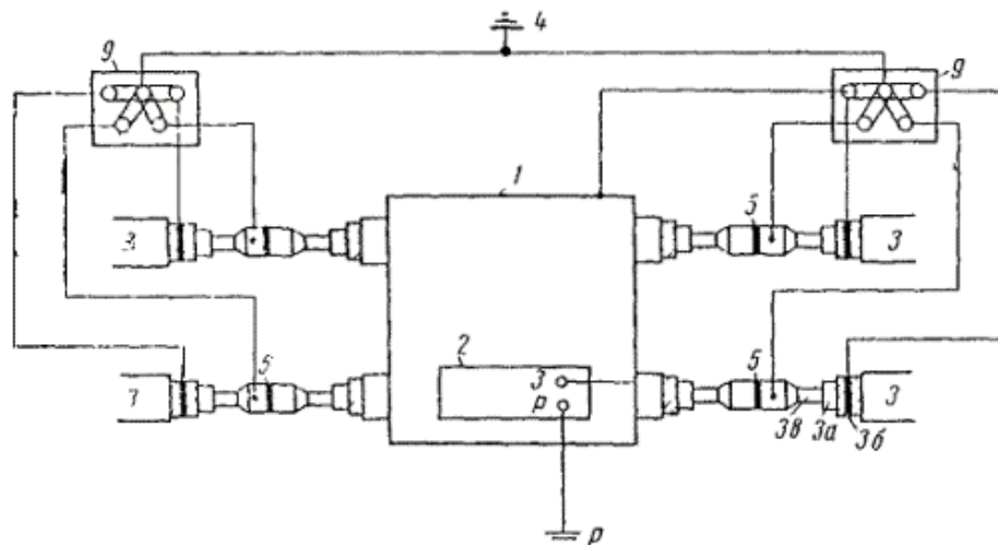
Рис. 11.8. Ввод в НУП и заземление кабелей с изолирующим покрытием ( r_3 \leq 300 \text{ Ом*м} )
