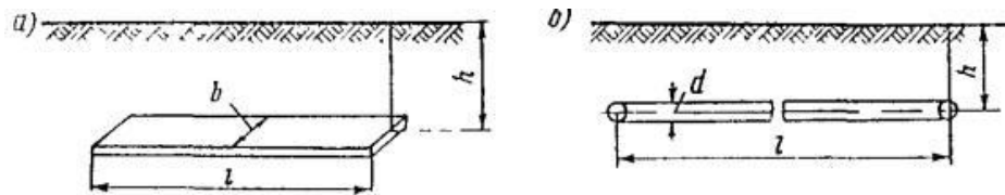
Рис 2.5. Протяженные заземлители: а) полосовые; б) цилиндрические
