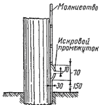
Рис 3.2 Устройство молниеотвода с искровым промежутком
