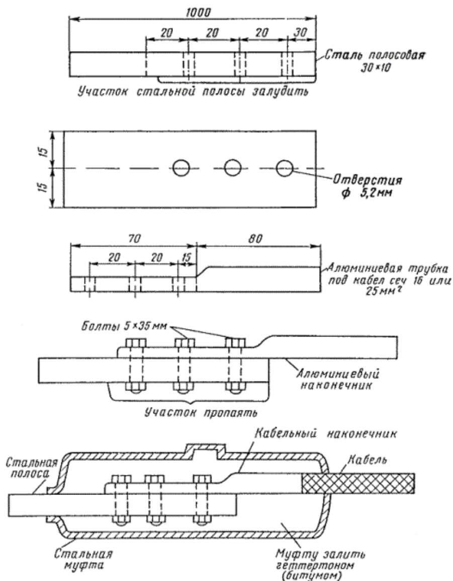
Рис.5.3. Устройство стыка стальной полосы и наконечника
