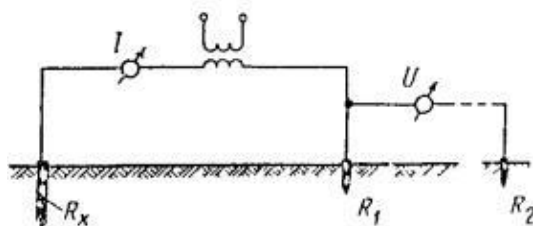
Рис.8.8 Схема измерения сопротивления измерительного (вспомогательного) заземлителя с помощью амперметра -вольтметра
