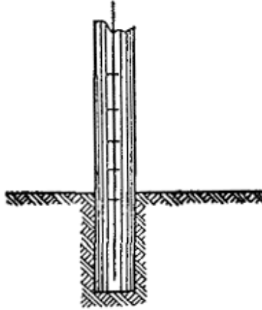
Рис. 3.3. Заземление молниеотвода вдоль комельной части столба
