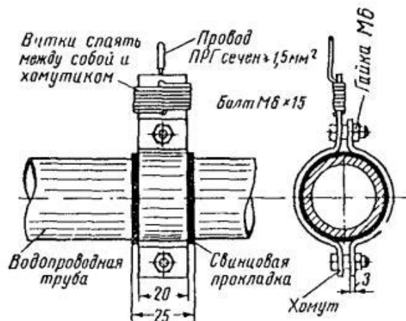
Рис.4.2. Устройство заземления у абонентского пункта СТС
