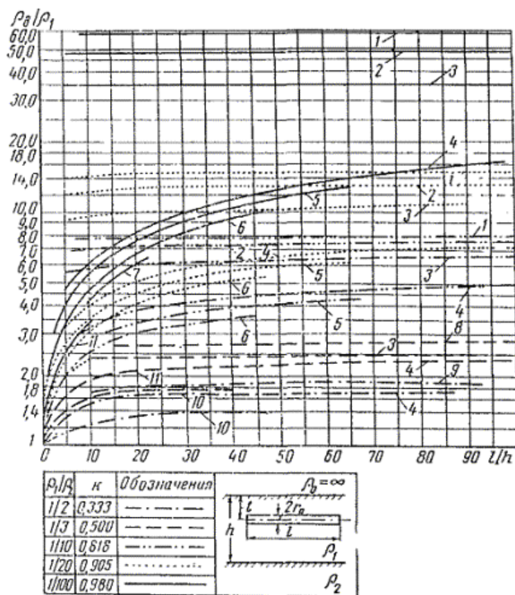
Рис.2.12. Графики значений действующего удельного сопротивления грунта для горизонтальных заземлителей при различных отношениях t/h и k > 0 :
