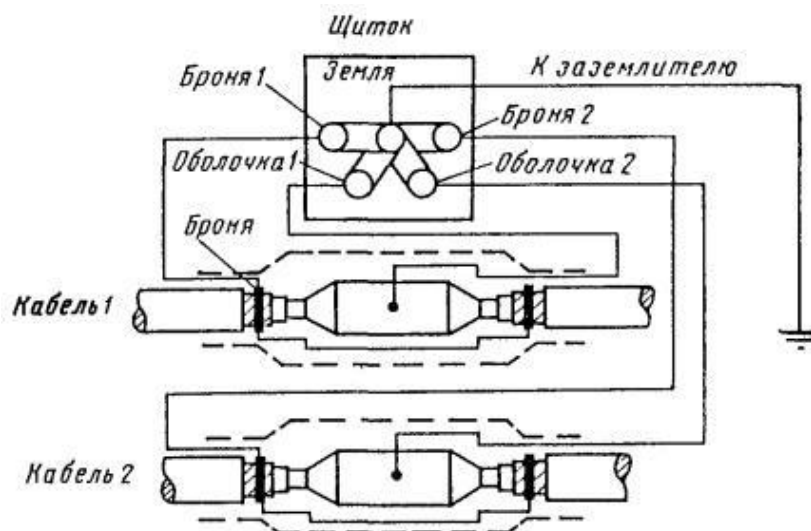
Рис.11.2. Схема соединений КИП-2 для бронированных кабелей с изолирующим покровом
