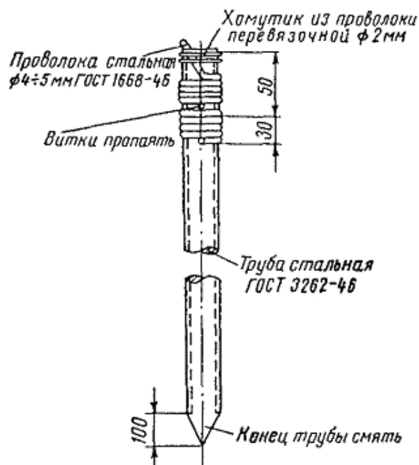
Рис.3.7. Устройство заземления из одной трубы
