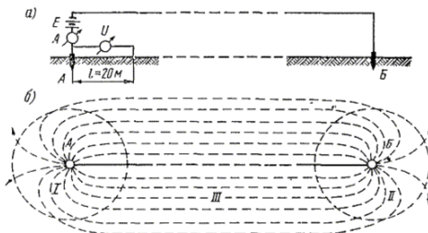
Рис.1.1. Схема измерения сопротивления заземления (а) и поле токов в земле (б)
