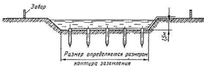
Рис.7.1. Устройство контура заземления на дне пруда
