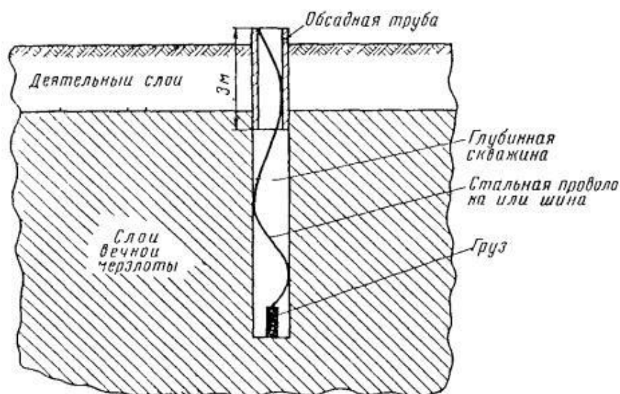
Рис.3.13 Устройство глубинных заземлений в районах вечной мерзлоты
