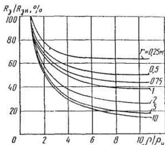
Рис.2.22 Относительное снижение сопротивления заземления в случае применения насыпного грунта при различных радиусах выемки
